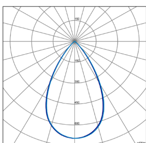
NT28/OPT-30°-2850-64W
