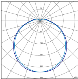
LUNA/F-280-IP65-18W
