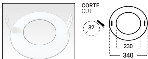
ACCESORIO CIRCULAR PARA TECHO DE PLADUR CIRCULAR FRAME RECESSED MOUNTING
