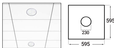
ACCESORIO CUADRADO PARA TECHO DE PERFILERIA VISTA SQUARE FRAME RECESSED MOUNTING
